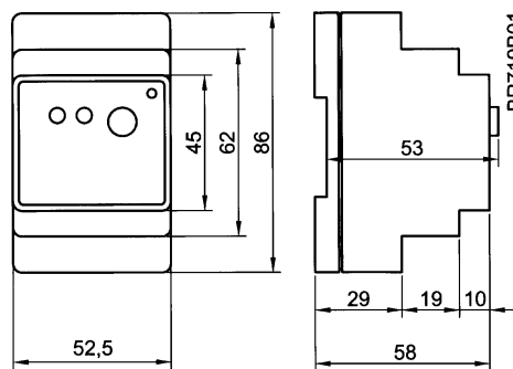
Размеры ETN (мм)
