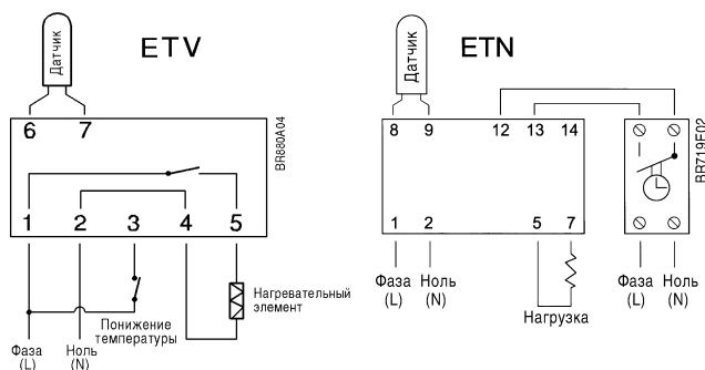
Подключение ETV
